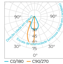
Gráfico 3 – Neu 2 | Balizador de Sobrepor STH8750/30
