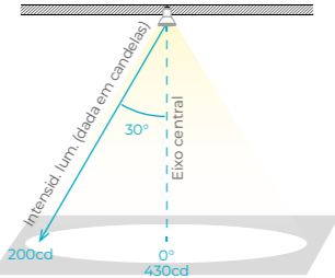
Ilustração 2 – MR16 ECO STH8538/30
