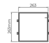
Dimensão do corte: 245x245mm
