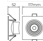
Dimensão do corte: Ø90mm (3,5/8")
