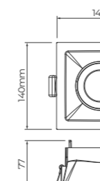
Dimensão do corte: 127x127mm
