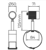
Diâmetro máximo da cinta: Ø130mm
