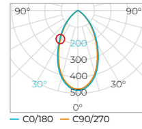
Gráfico 2 – MR16 ECO STH8538/30
