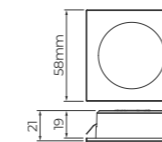
Dimensão do corte: Ø50,8mm (2")
